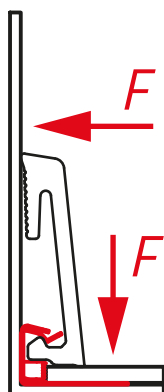
Opcja 1. (w trakcie kładzenia podłogi) Specjalny klips beznarzędziowy ze stali nierdzewnej
