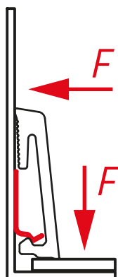
Opcja 2. (do gotowej podłogi) Plastikowy klips na wkręty
